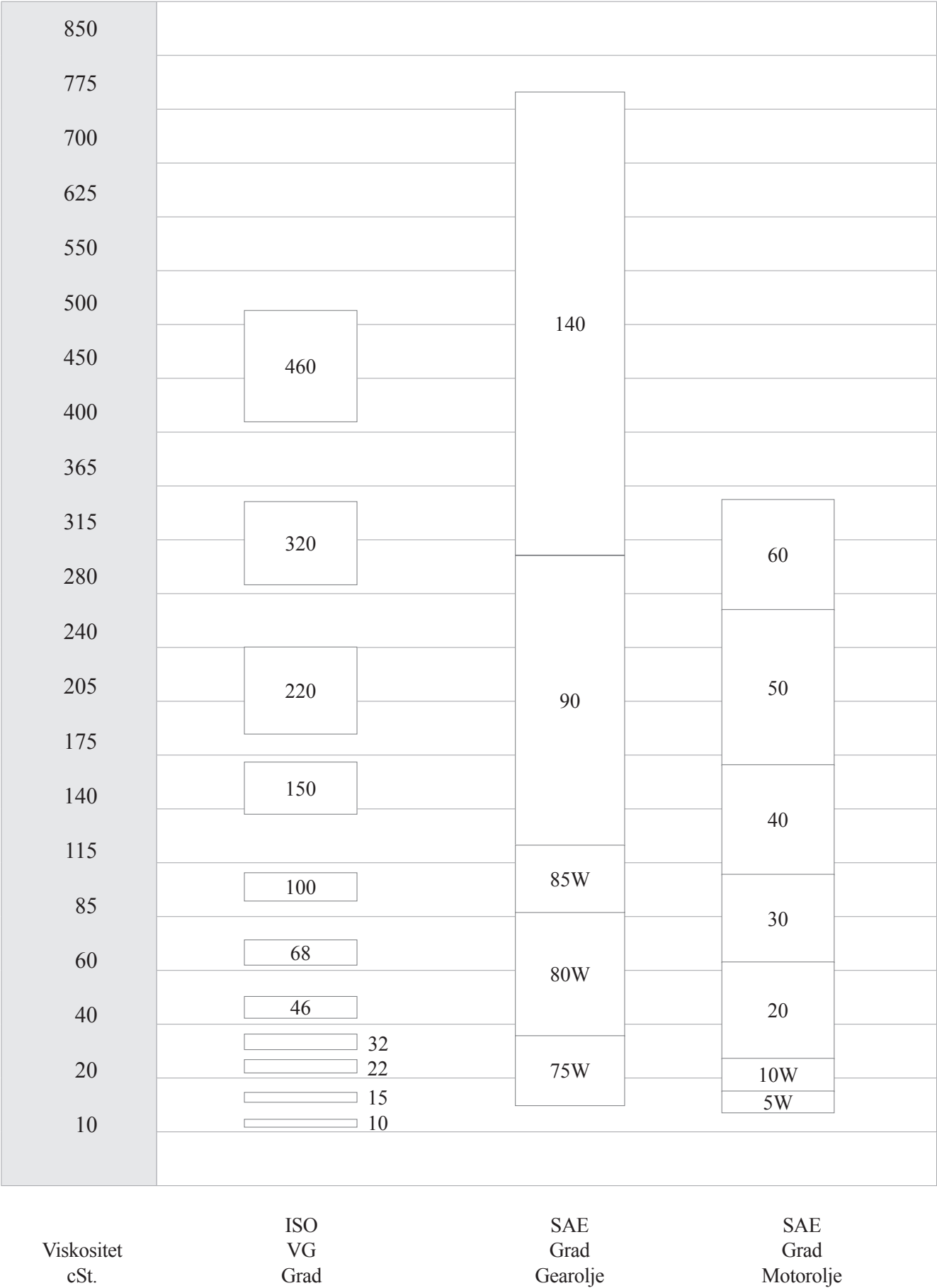
SAMMENLIGNING MELLOM ISO-KLASSER OG SAE-GRADER
